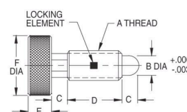
Radiused Delrin® Plunger
